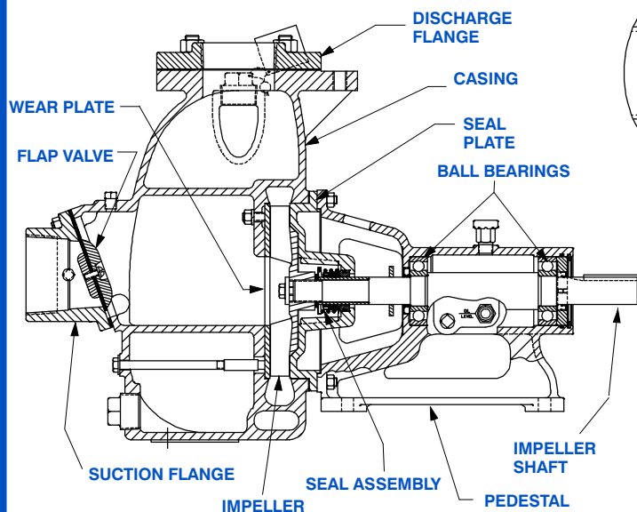
83C3-B SHOWN
