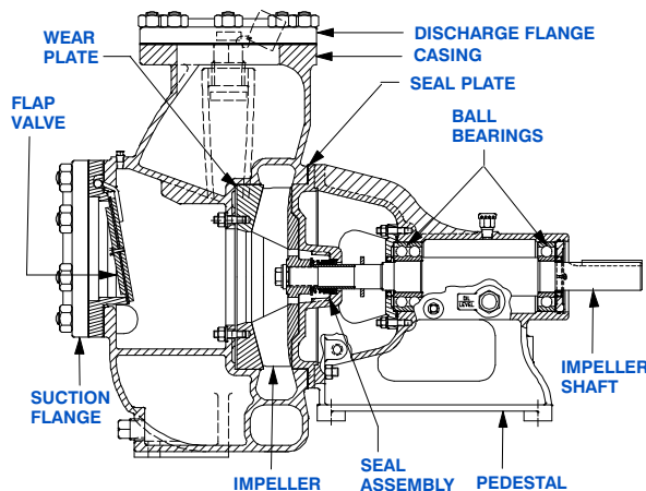
88A52-B SHOWN
