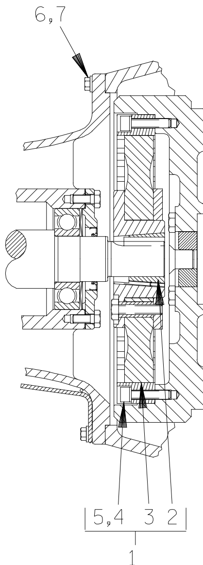
44162—119 Drive Assembly
